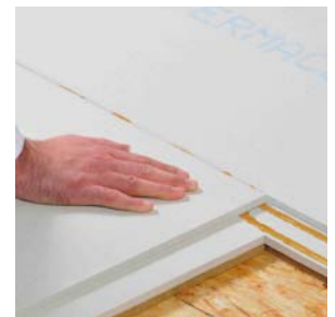
Verlijmen van de vloerelementen onderling met volledig met lijm gevulde liplas.
