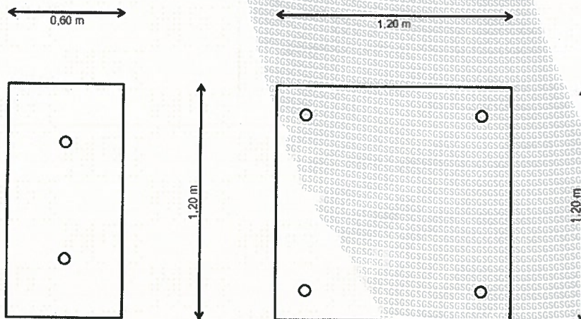
Figuur 3: Bevestigingspatronen Therma ™ -systeem niPIR-N
