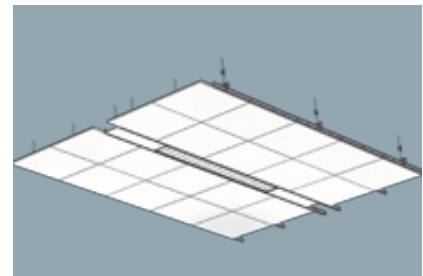
Verdekt uitgevoerd systeem met inleg-armaturen op zichtbare Quick-Lock draagprofielen
