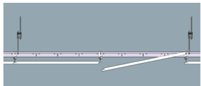
Cross-Lock systeem met opwaarts uitneembaar paneel
