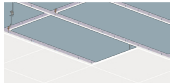
Cross-Lock systeem met opwaarts uitneembaar paneel
