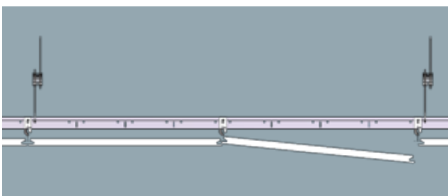
Cross-Lock systeem met neerwaarts uitneembaar paneel
