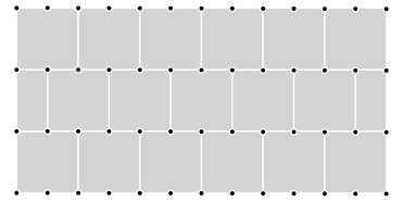
600 x 600 half steensverband
